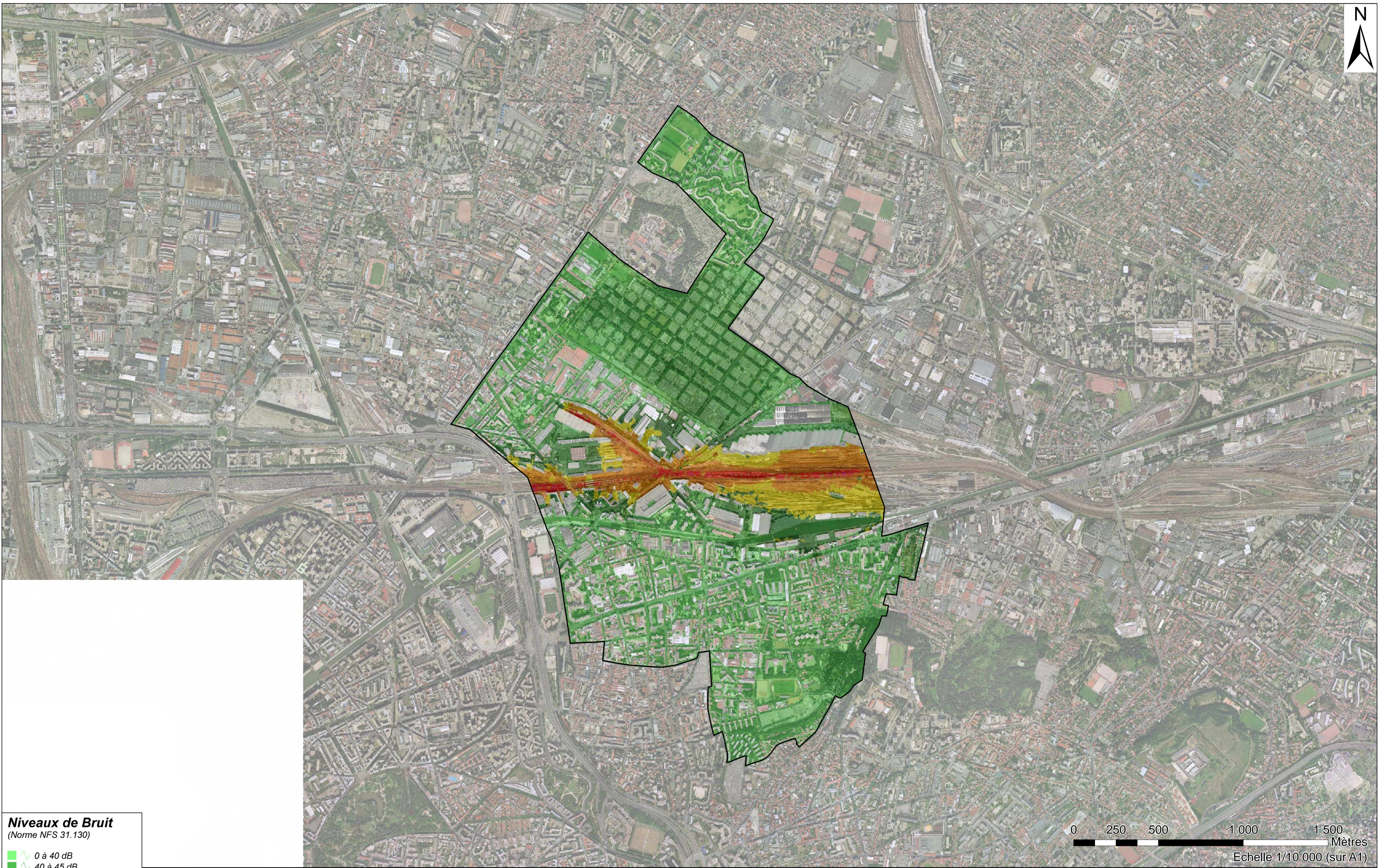
Carte de bruit Commune de Pantin Isophone fer valeur "Lnight"
